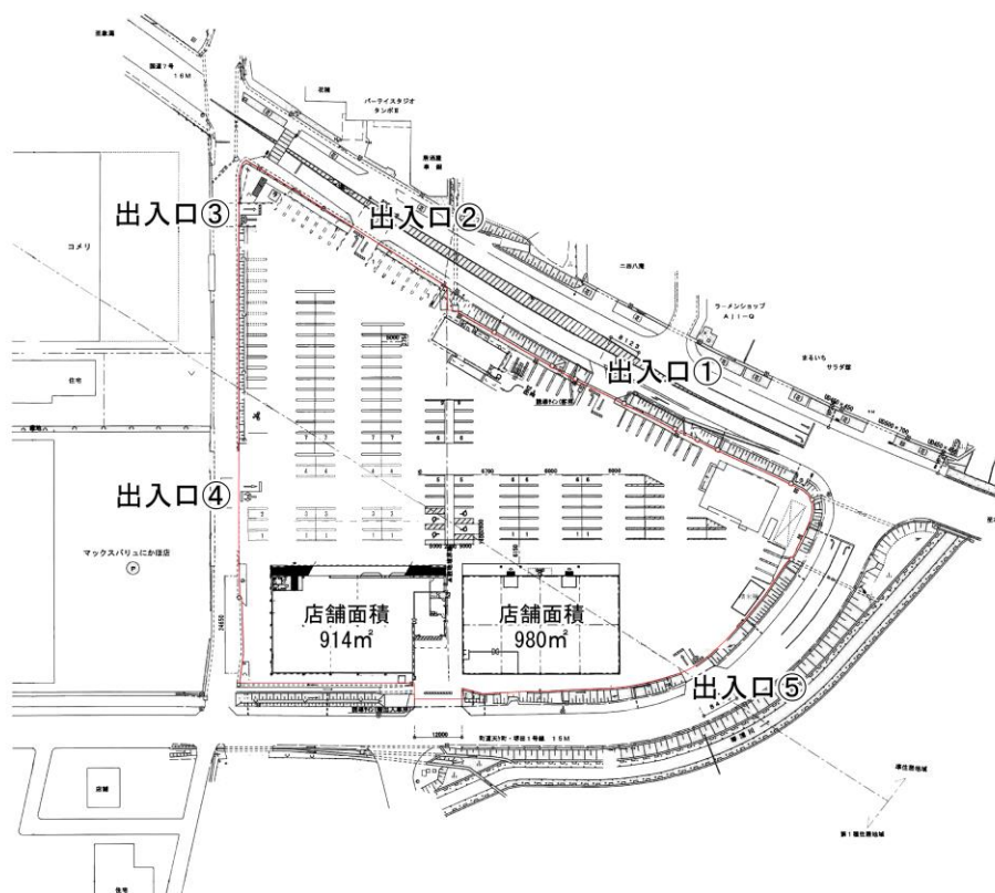
建物配置図及び 1 階平面図 (変更後)
